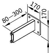
Distanziatore per supporto a parete 71813.
