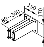
Distanziatore per supporto a parete 70867.
