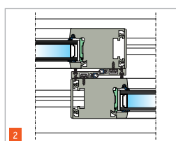
porta-finestra alzante scorrevole in PVC con elemento laterale fisso
