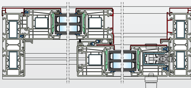
sezione orizzontale della porta alzante scorrevole KAB 908: forme assolutamente simmetriche
